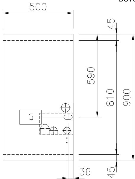
Boven aanzicht
